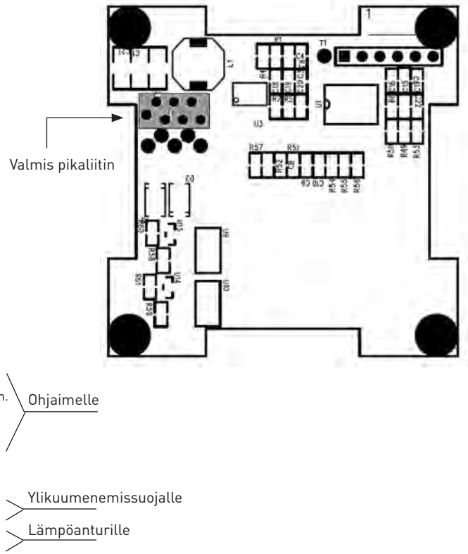
Ohjainkortin kytkentä ohjaimessa
